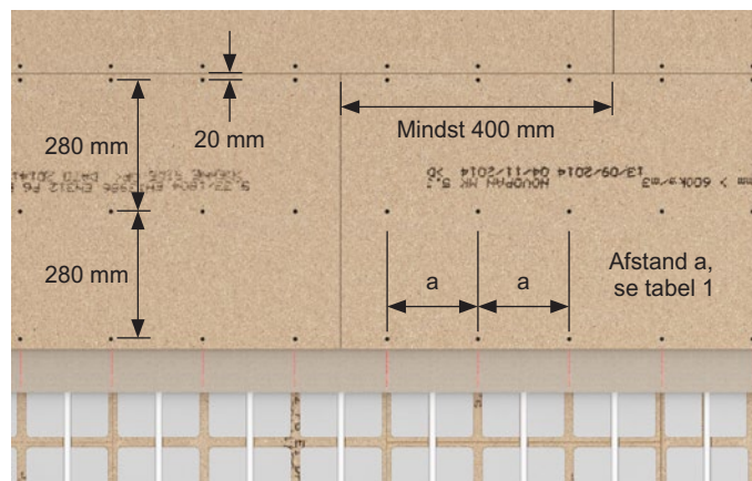
Figur 2 Mellemlagsplader på 22, 25 og 38 mm Novopan Klimagulv – skrueafstande og forskydning af pladestød.
